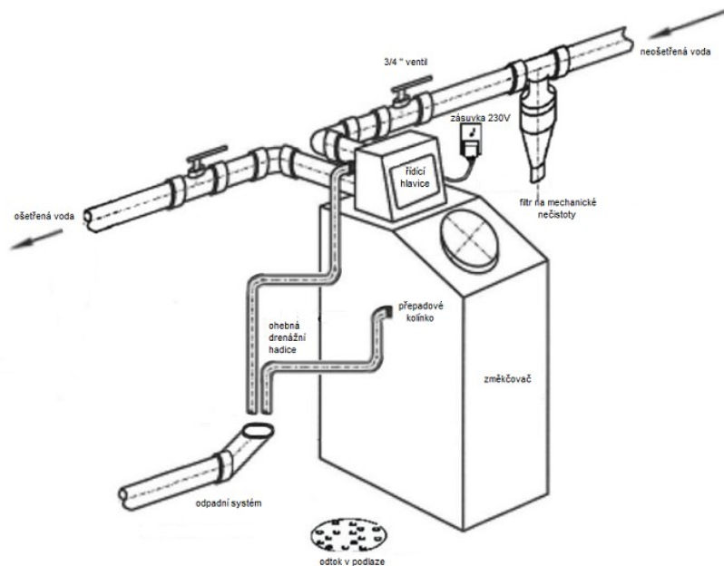
obrázek 1 – Instalační plán
