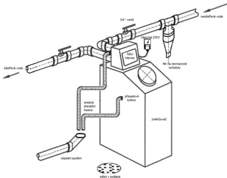
obrázek 1 – Instalační plán
